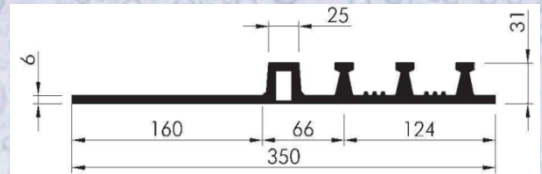
AM 350 o parte neteda Elastoflex® conform DIN 7865, Parte 2
