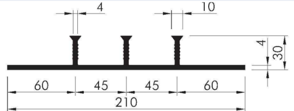
Colier racord conform Modul 853.4101 SA 210
