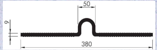
Omega 380 cu material incorporat Elastoflex® conform DIN 7865, Parte 2
